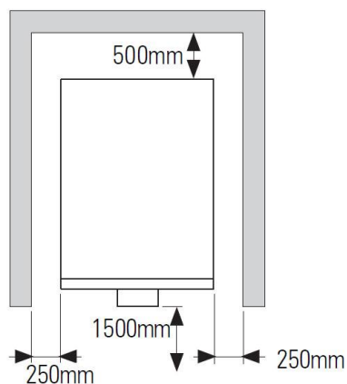
Рисунок 1.16 Минимальные расстояния для установки
