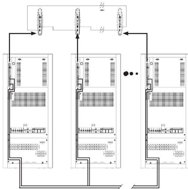
Рисунок 3.6 Пример подключения коммуникационной шины параллельной системы
