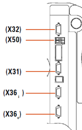
Рисунок 1.10 Разъемы интерфейсов
