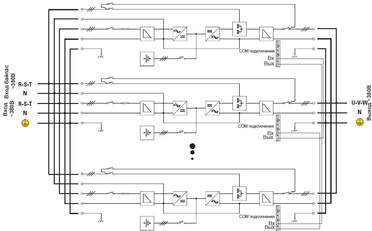
Рисунок 1.14 Однолинейная схема параллельной работы ИБП с отдельным входом статического байпаса
