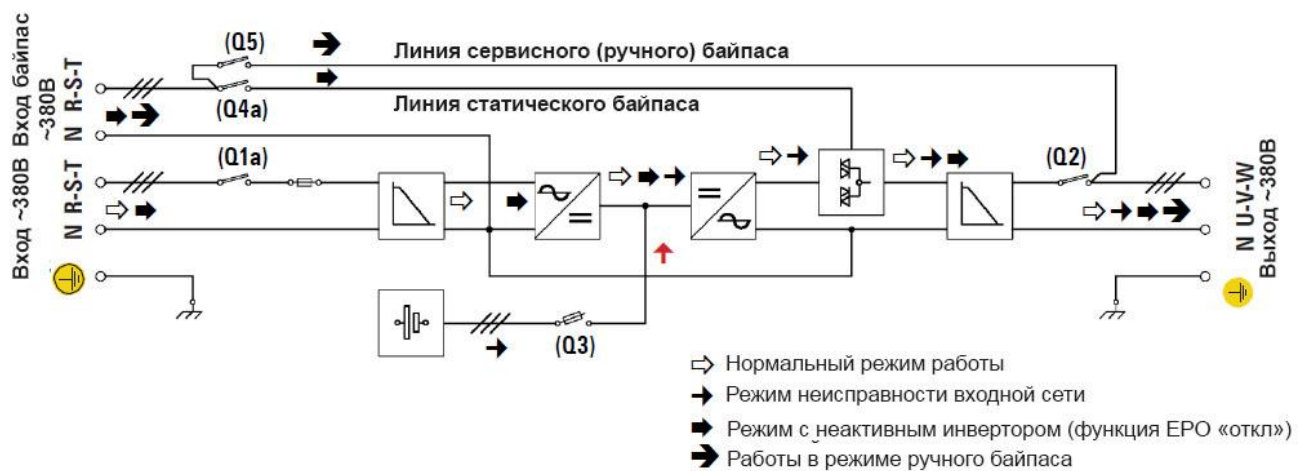
Рисунок 1.11 Однолинейная схема ИБП
