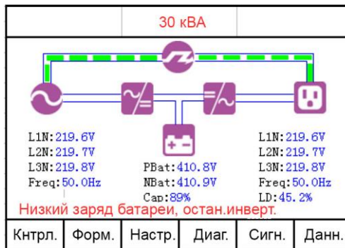
Рисунок 5.2 Экран 0.0 главного меню
