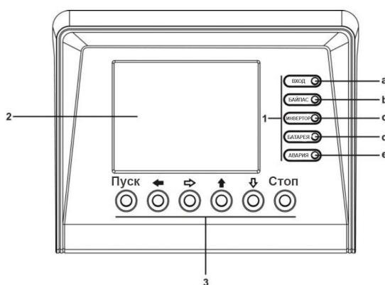
Рисунок 1.2 Панель управления
