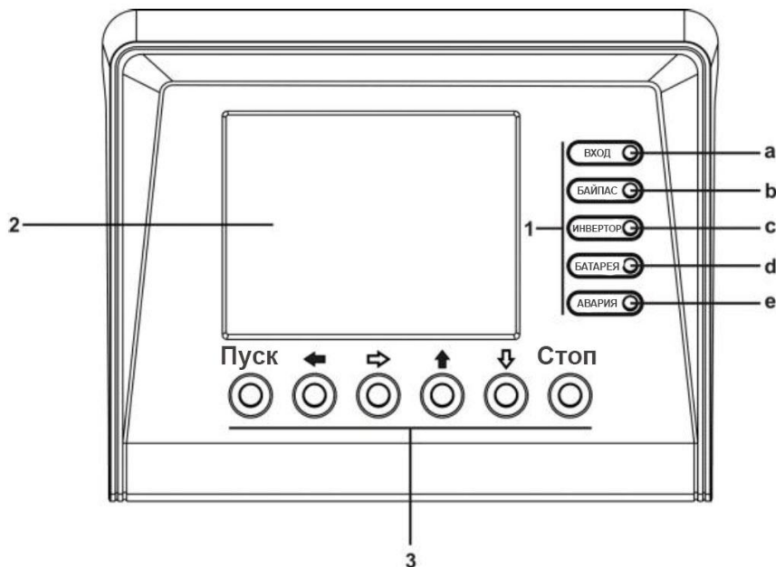
Рисунок 5.1 Внешний вид панели управления
