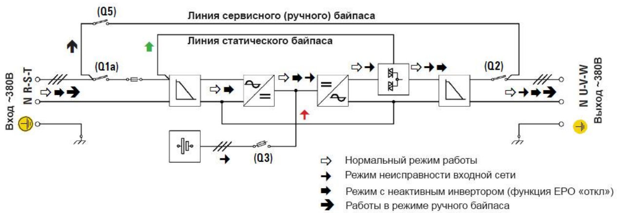
Рисунок 1.11 Однолинейная схема ИБП
