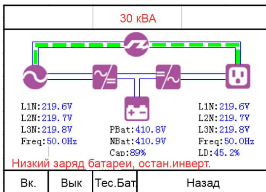
Рисунок. 5.3 Экран 1.0 меню контроля
