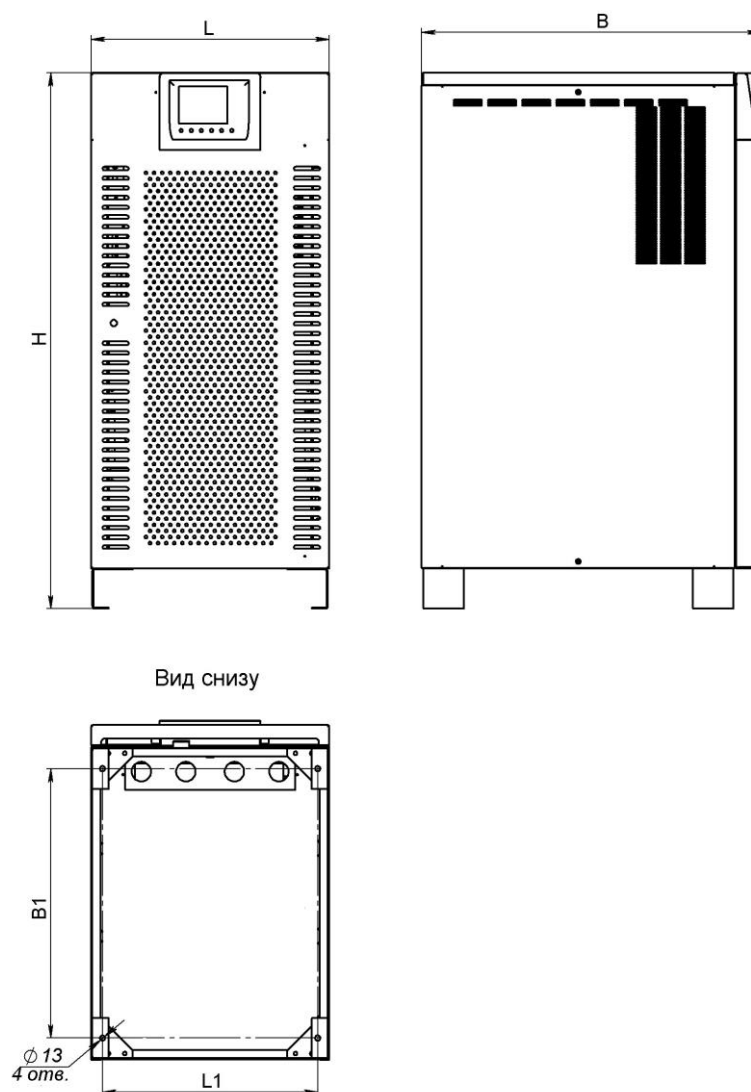
Рисунок 1.15 Габаритный чертеж ИБП
