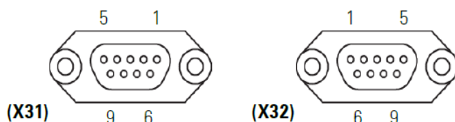
Рисунок 3.4 Расположение контактов разъема DB9 (X31) и (X32)
