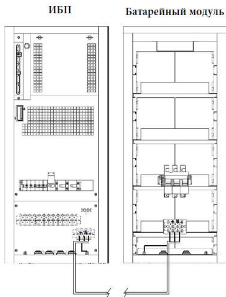
Рисунок 3.1 Подключение к ИБП батарейного модуля
