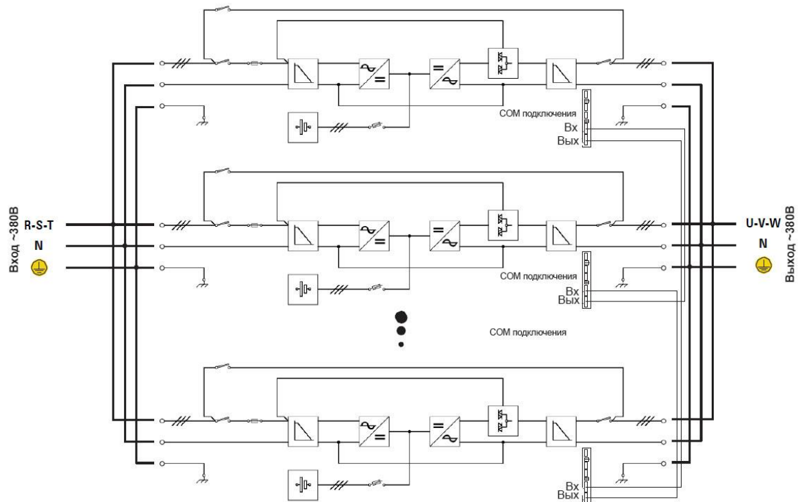
Рисунок 1.13 Однолинейная схема параллельной работы ИБП
